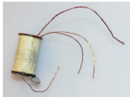
Der Spulendraht ist durch Lack isoliert. An den Enden entfernt Jahn die Schutzschicht und verlötet die Spule mit dem Relais
